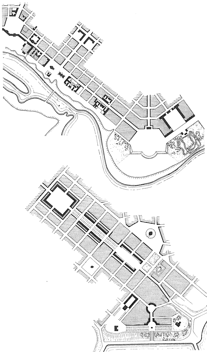
Рис. 155. Варианты регулярной планировки центров Николаева (1) и Одессы (2)
